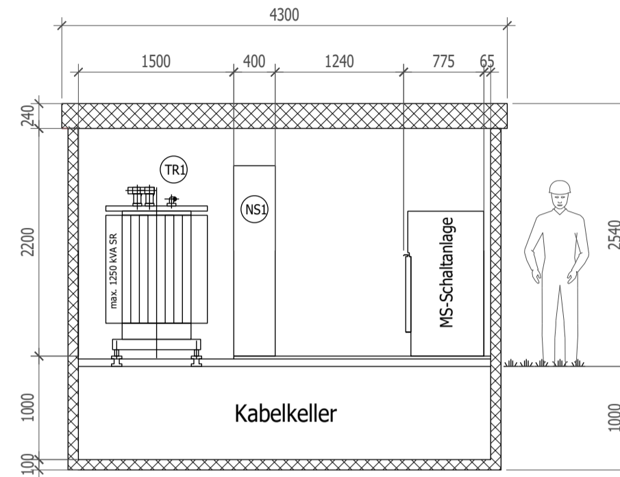
Schnitt B-B
